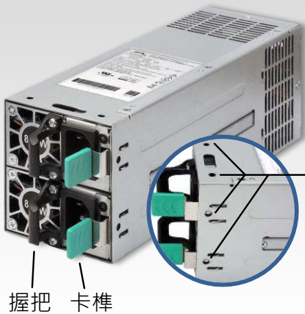
安裝孔 (8個)
